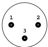
CONNETTORE DMX, DISPOSIZIONE CONTATTI VISTA FRONTALE
