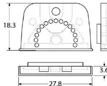
Tappo End cap
